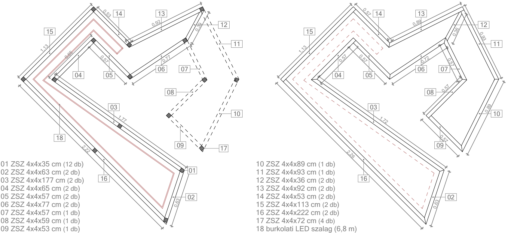
kiterített homlokzat
